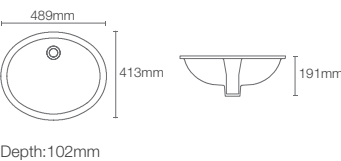
CANTON™ | K-2210IN-0
