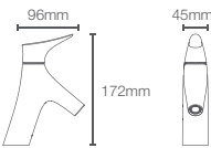
VIVE | K-23968IN-4-CP
