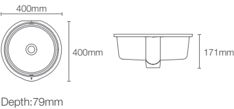
VERTICYL™ | K-2883IN-0
