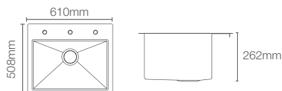
STRIVE™ K-38795IN-NA
