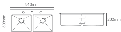
STRIVE™ | K-38802IN-NA
