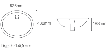
CANTON™ | K-2211IN-0
