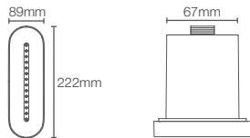
STATEMENT™ K-26300IN-CP
